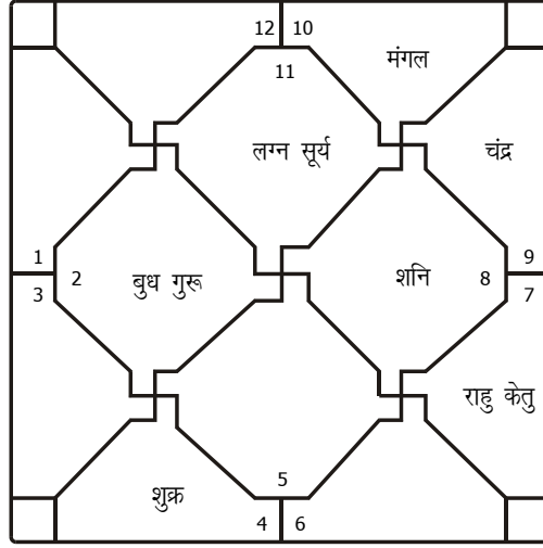
विशांश
