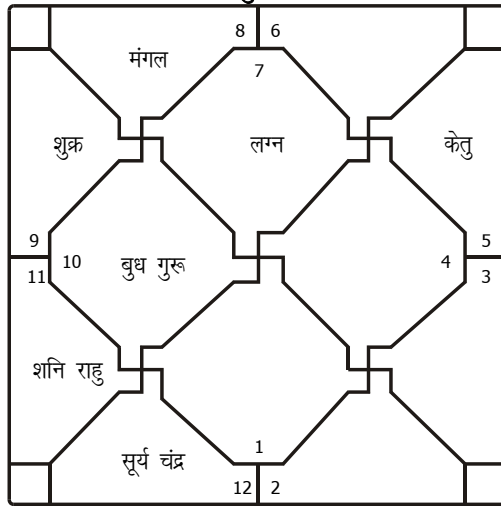
चतुर्थांश
