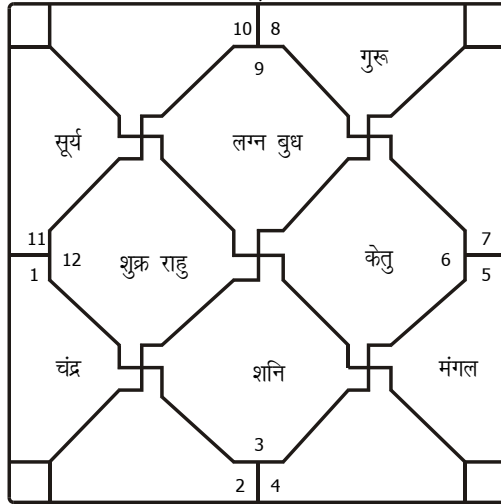
षष्ट्यंश
